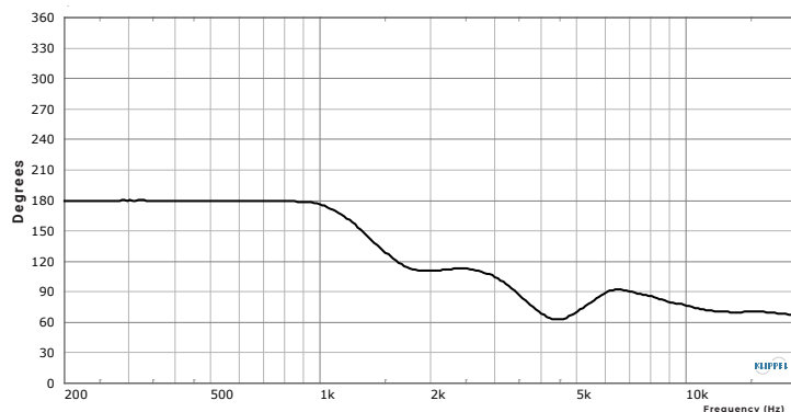
Beamwidth
